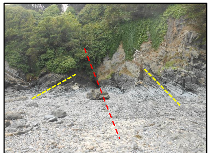
Fig.96 : Fracturation (F) et plissement de la formation de Binic
