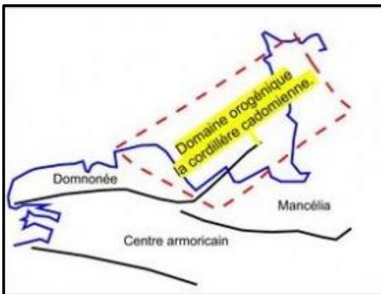
Fig.1 Extension de la chaîne cadomienne
