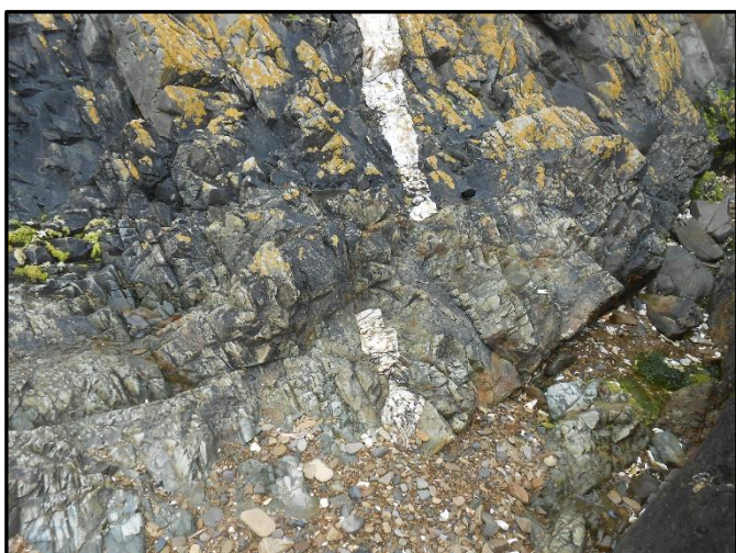
Fig.105 : Faille décalant un filon de quartz
