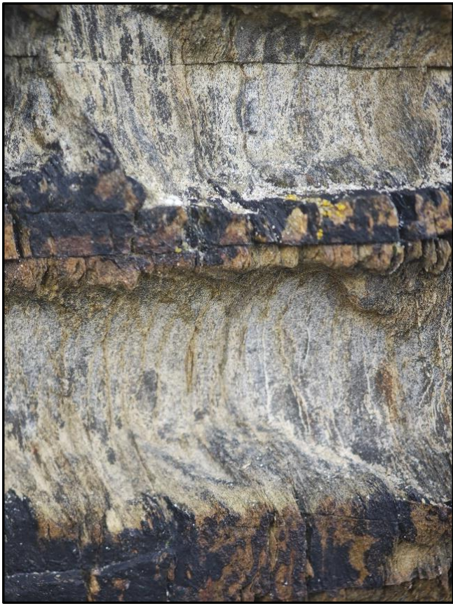
14 : Kink-bands ( ?) dans une formation sédimentaire
