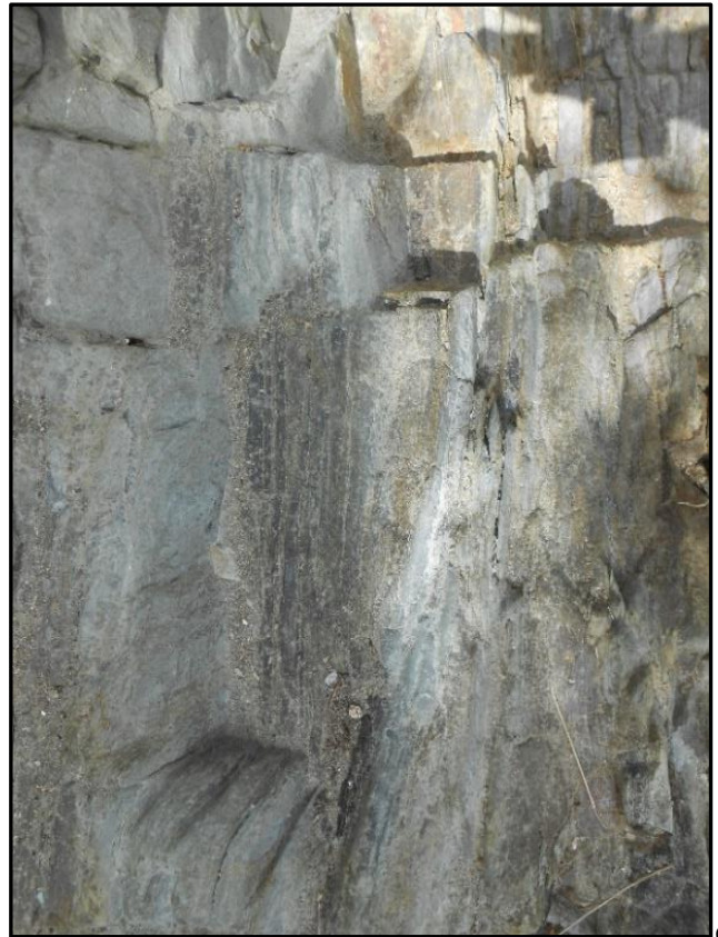
17 : Formation schisteuse bleue (?) d'Illemont
