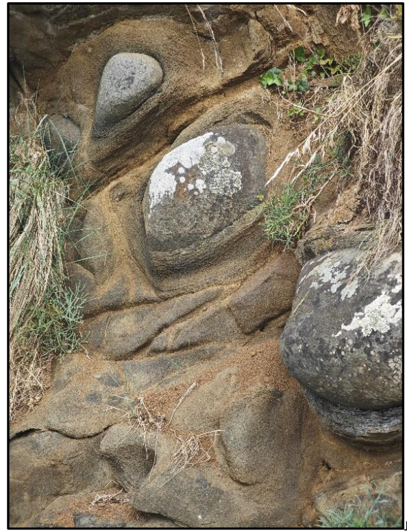
29 : Altération en boules de la dolérite
