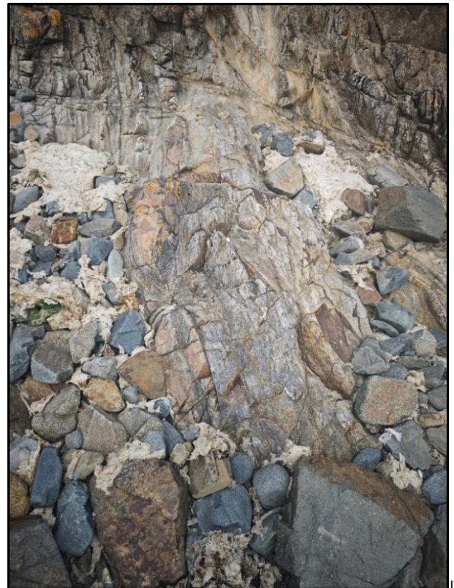
31 : Pillow-lavas ?
